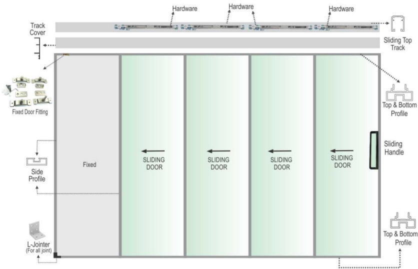
HLX -44 1 Fix + 4 Sliding Door
